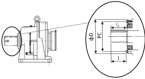
甲板防水形 サイクロ減速機防滴部寸法
