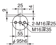
断面a-a
