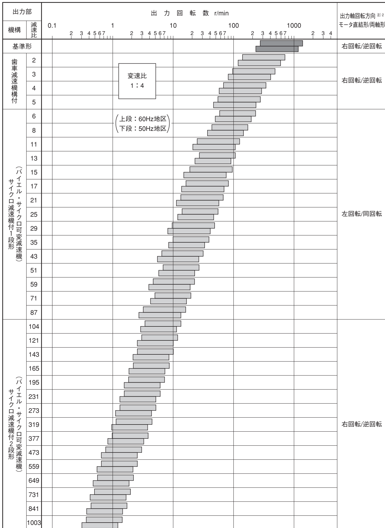
■A形B形出力回転数範囲、出力軸回転方向
