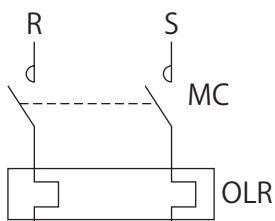
図E30 単相モータ：0.1～0.4kW（コンデンサ始動コンデンサ運転形）
