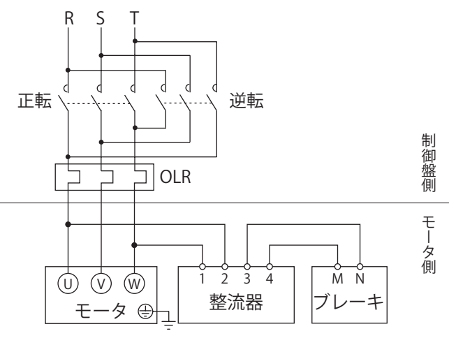
図E36 三相モータ : 0.55kW プレミアム効率三相モータ : 0.75~3.7kW 高効率三相モータ : 0.4kW FB-1D, FB-1E~FB-5E
