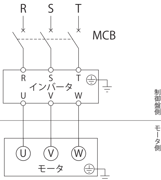
図E28 三相モータ 三相モータ : 0.1～0.55kW プレミアム効率三相モータ : 0.75～3.7kW インバータ用三相モータ : 0.1～0.4kW インバータ用プレミアム効率三相モータ : 0.75～3.7kW 高効率三相モータ : 0.2～0.4kW
