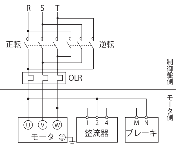
図E35 三相モータ : 0.1~0.4kW 高効率三相モータ : 0.2kW FB-01A1~FB-05A1
