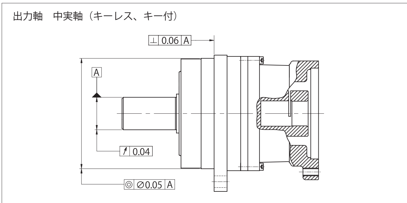
図 C7 中実軸機械的位置精度
