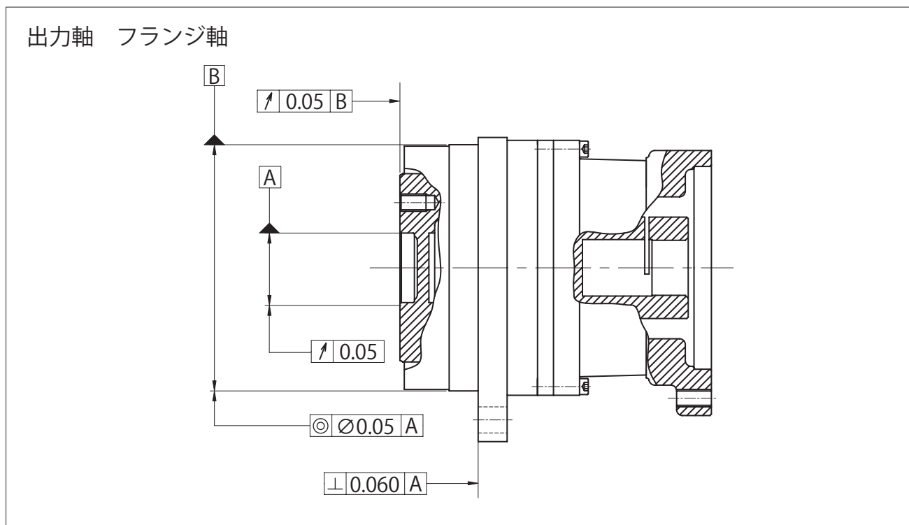
図 C8 フランジ軸機械的位置精度
