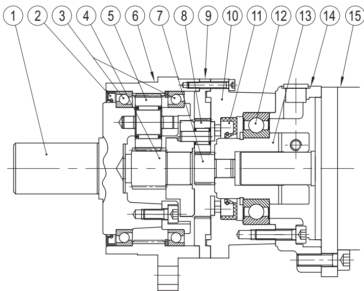
図 C1 2 段形 (例: ANFX-P120N)
