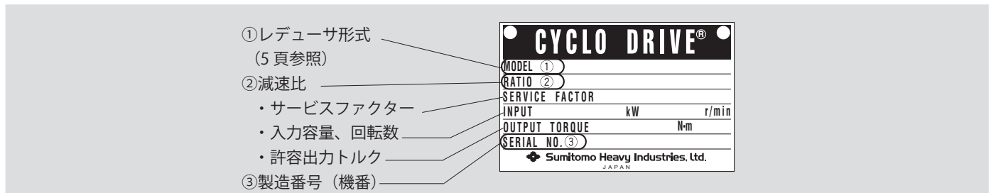
図2 銘板タイプ2
