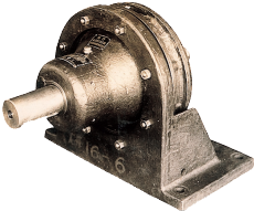
国産サイクロ試作 1 号機
