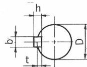
断面AA
