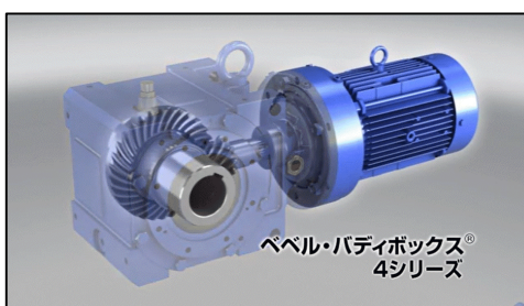
ベベル・パディボックス減速機
