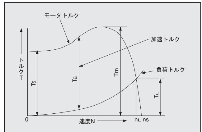
図 F9 トルク線図
