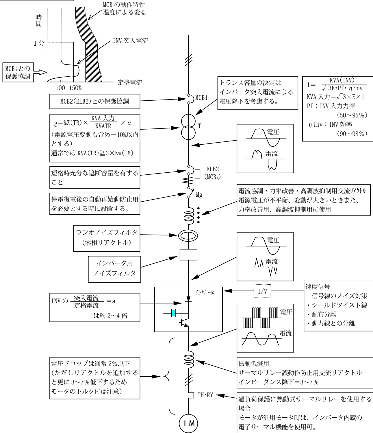
図 5 - 1 汎用インバータの入力及び出力電源系統
