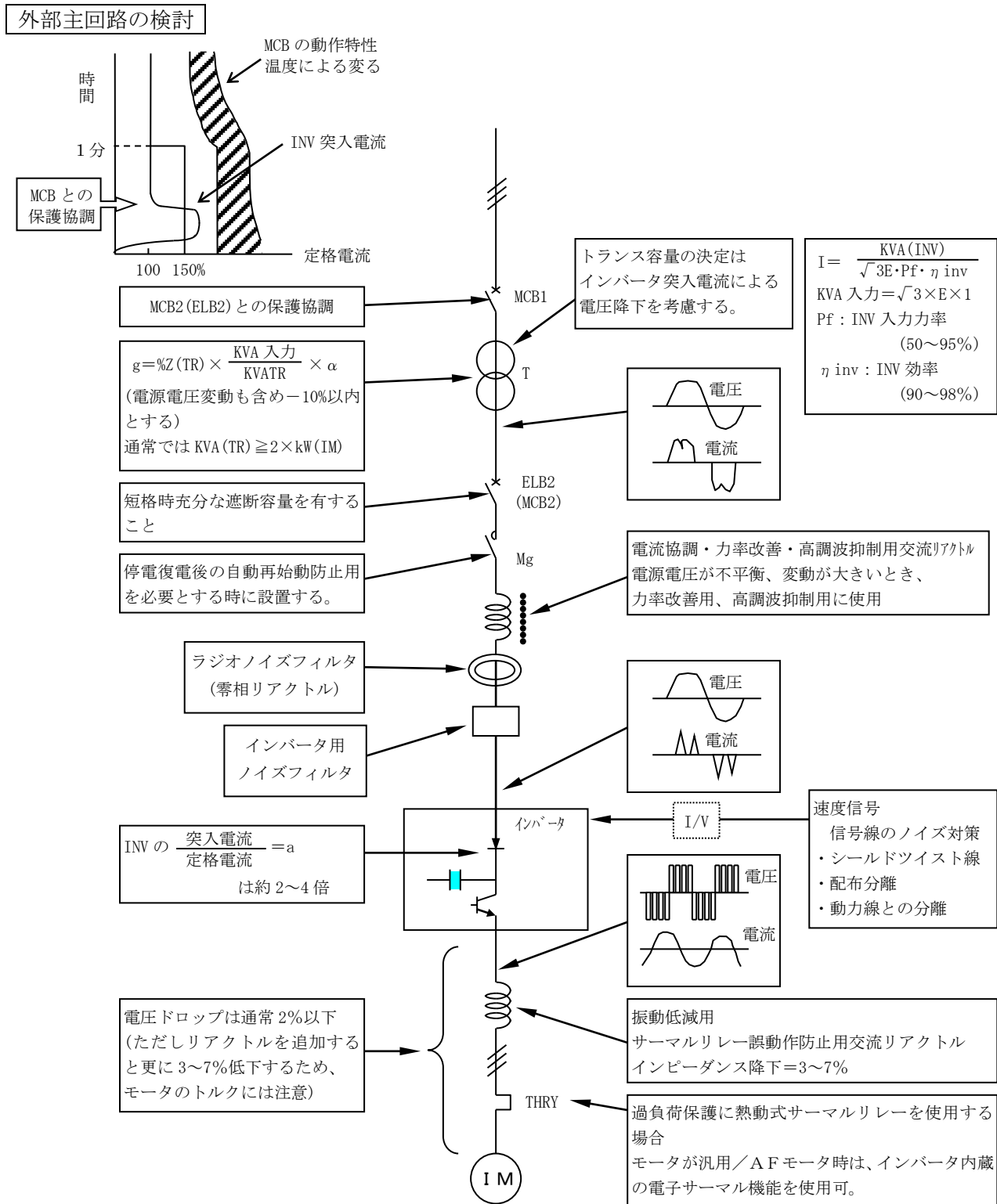
図 5-1 汎用インバータの入力及び出力電源系統
