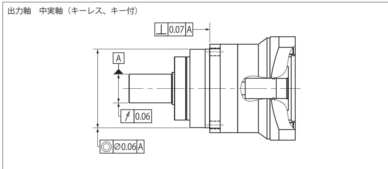
図 D7 中実軸機械的位置精度
