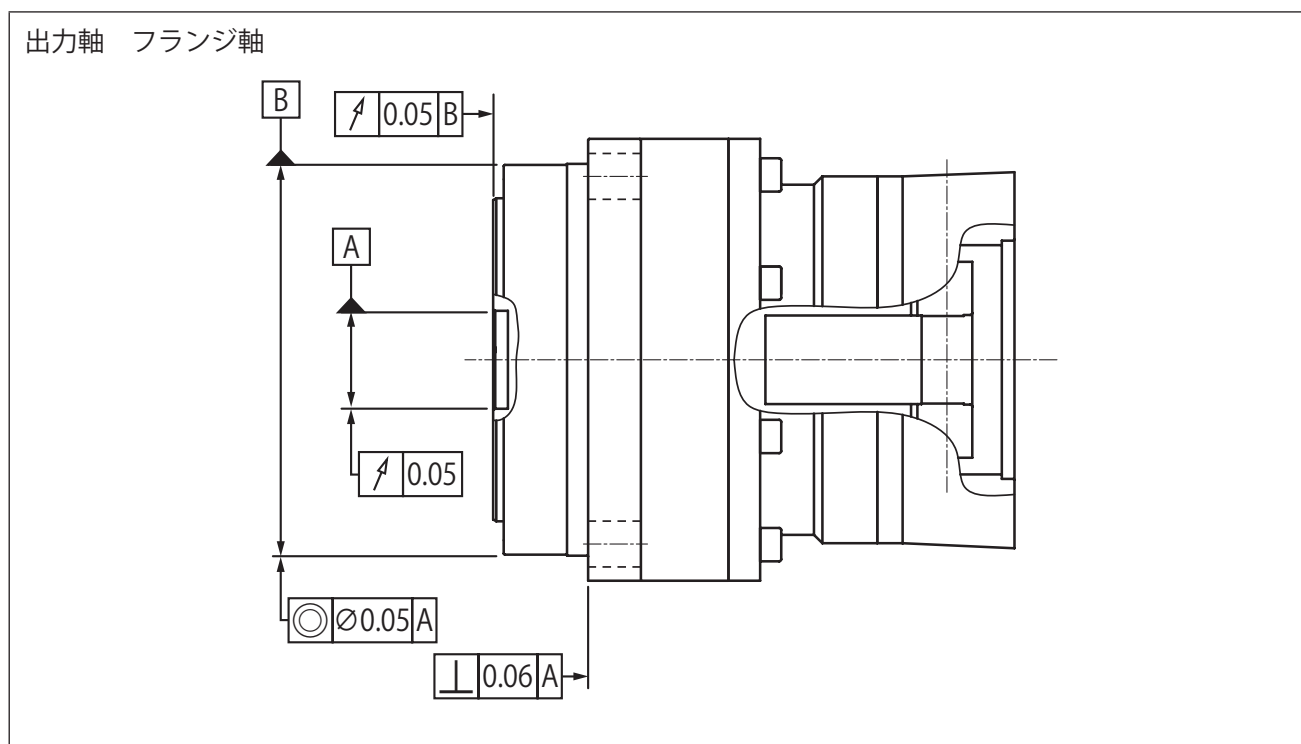
図 D8 フランジ軸機械的位置精度
