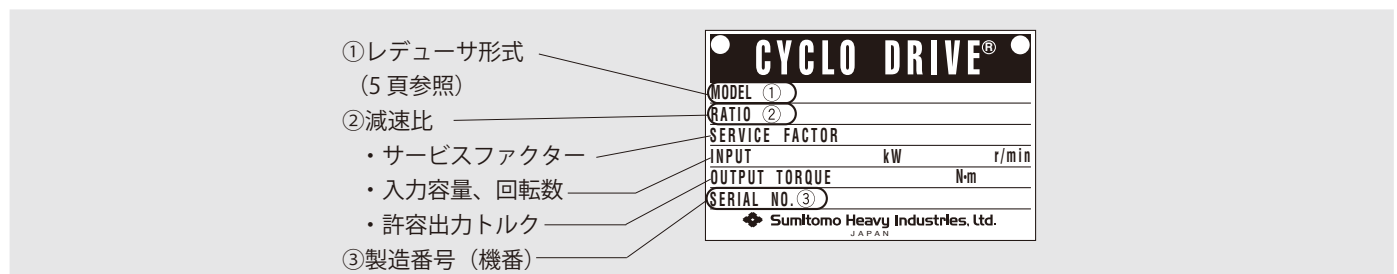
図 2 銘板タイプ2
