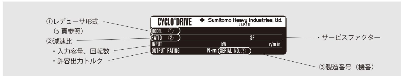
図 1 銘板タイプ1
