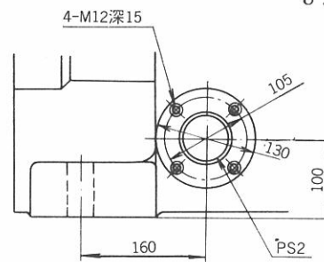
潤滑油出口詳細図
