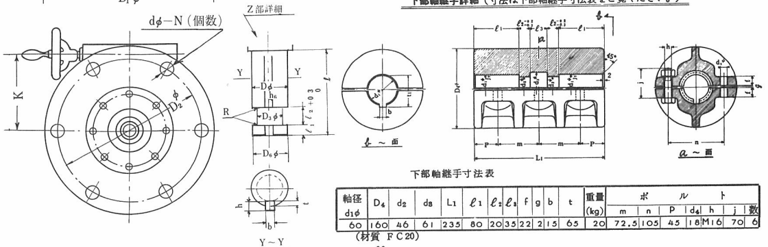
下部軸継手詳細 (寸法は下部軸継手寸法表をご覧ください。)
